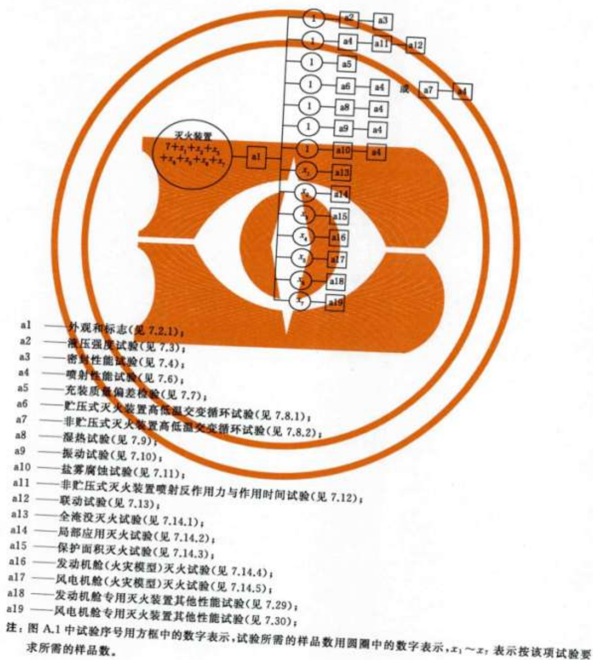
图 A.1 干粉灭火装置试验程序图
